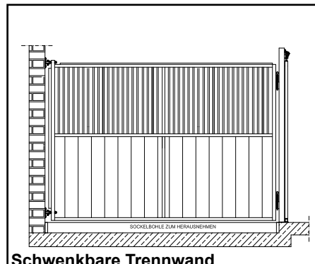
Schwenkbare Trennwand
