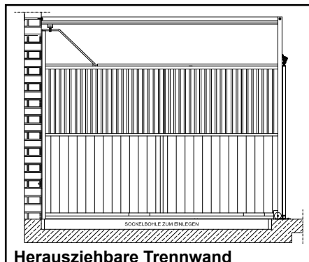
Herausziehbare Trennwand
