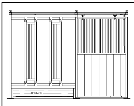
Vorderfront mit Sicherheits-Durchfressgitter & Schiebetür Holz/Gitter (Preis ab 1.204,- € + MwSt.)
