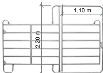
Panel mit Tor
