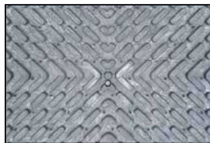
Unterseite mit Luftkanälen (kälteisolierend)
