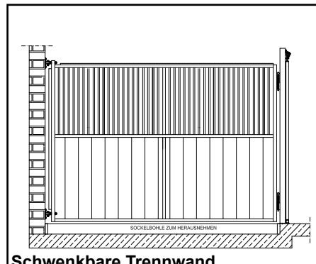
Schwenkbare Trennwand
