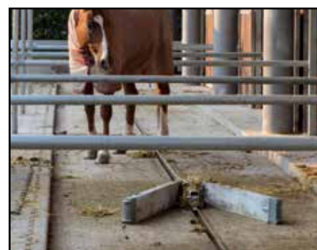
Entmistungsanlagen
