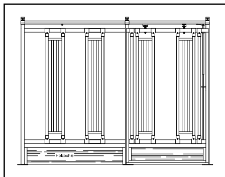
Vorderfront mit Sicherheits-Durchfressgitter & Schiebetür (Preis ab 1.385,- € + MwSt.)
