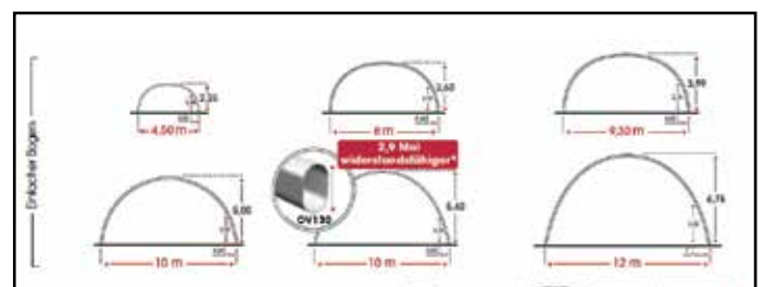
Maschinenhalle 12,00 m breit x 6,75 m hoch
