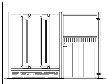
Vorderfront mit Sicherheits-Durchfressgitter & halbhoher Drehtür (Preis ab 1.330,- € + MwSt.)
