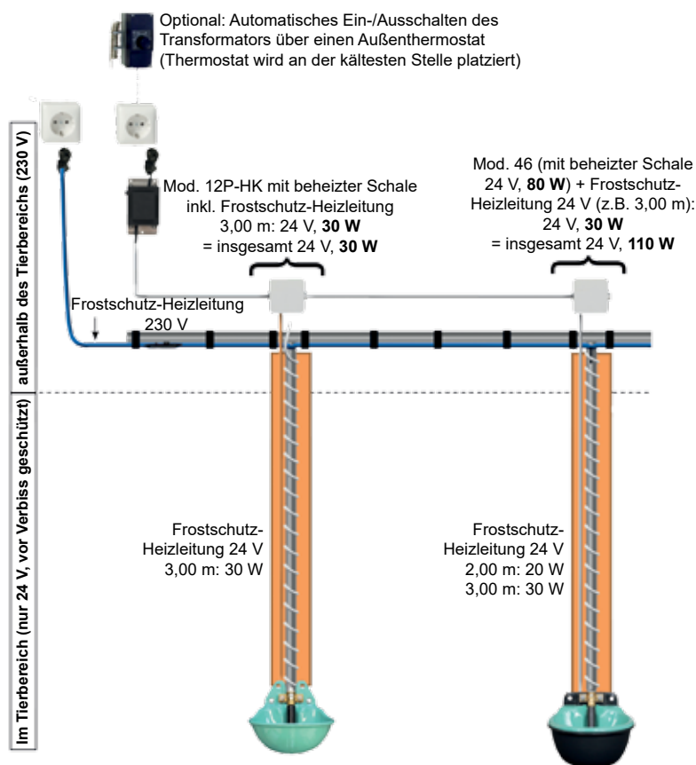
Aufbauschema mit optimierter Darstellung ohne Isolation der Rohre. Montageanleitung beachten.
