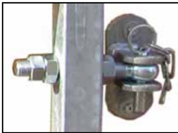
Massive, leicht verstellbare Aufhängung für alle Pfosten
