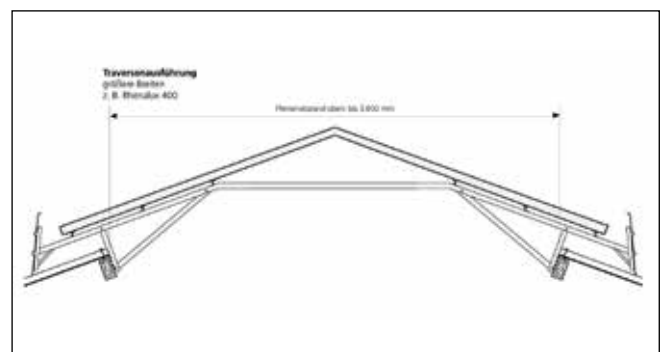
Traversenausführung größere Breiten z.B. Rhenalux 400
