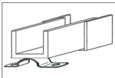
Mittenführungsschiene U 50/40/4
