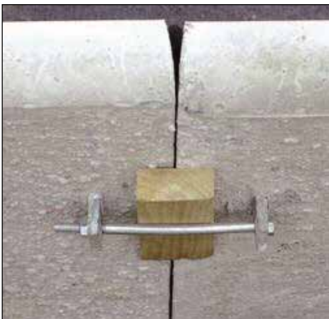
Verschraubung mit Holzkeil
