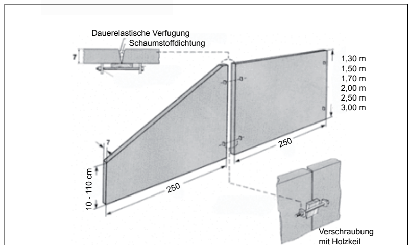
Stellrinne mit Traunsteiner Wandplatte
